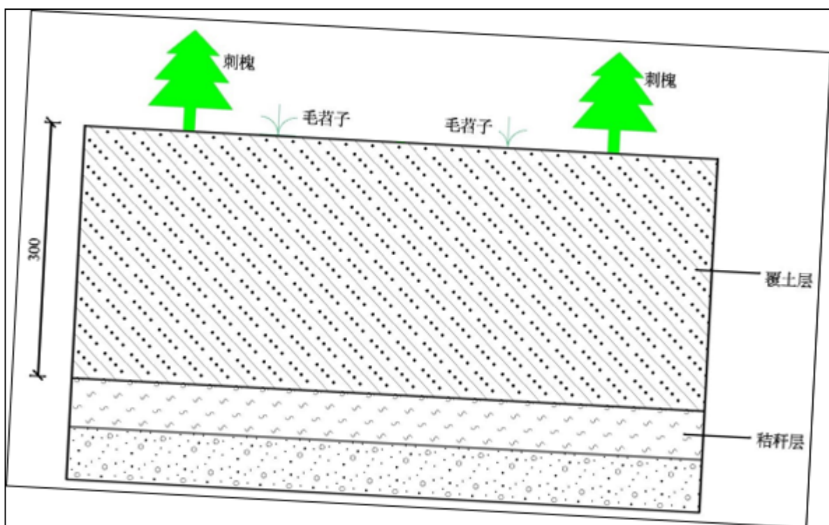
图 5-8 排土场土地复垦设计大样图
