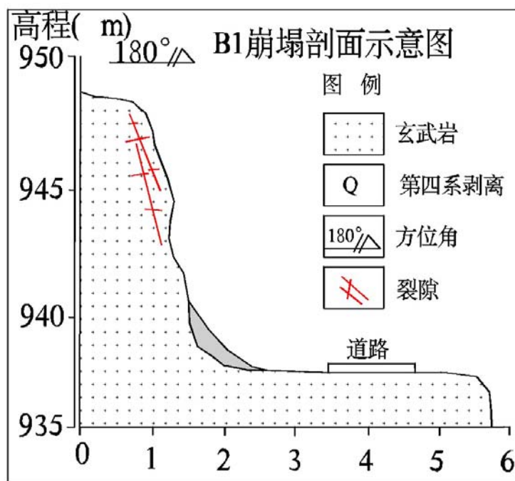
图 3-1 B1 崩塌隐患点剖面
