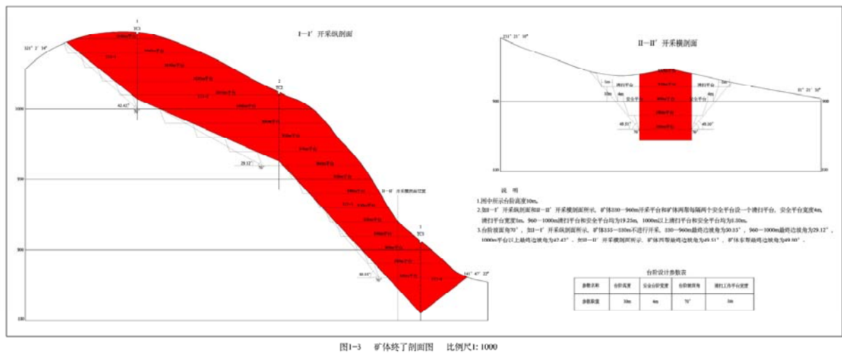
图 1-3 开采剖面
