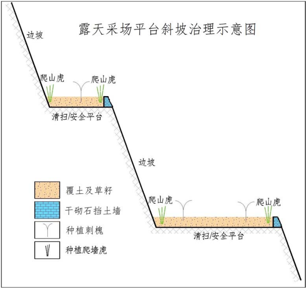
图 5-3 露天平台+斜坡复垦设计图
