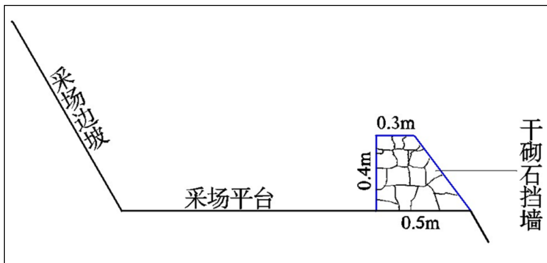
图 5-5 干砌石挡墙设计大样图
