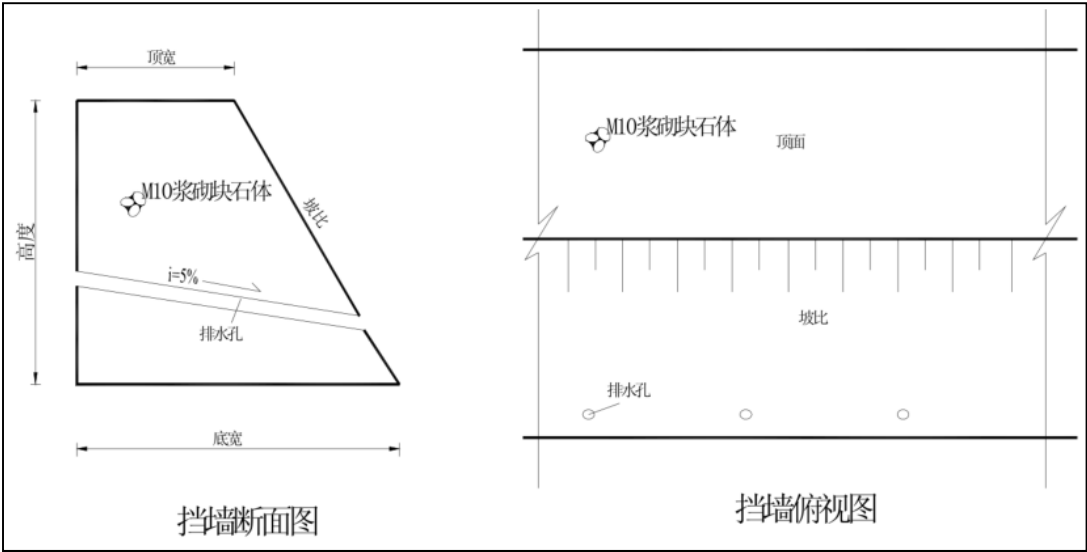
图 5-1 挡渣墙设计大样图
