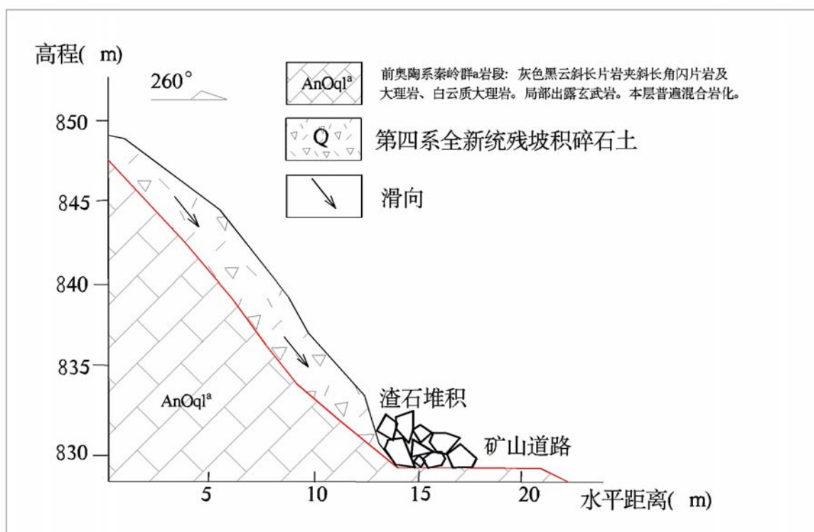
图 3-4 H1 滑坡隐患剖面图
