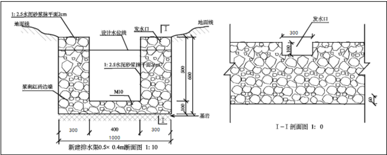
图 5-2 排水渠设计大样图
