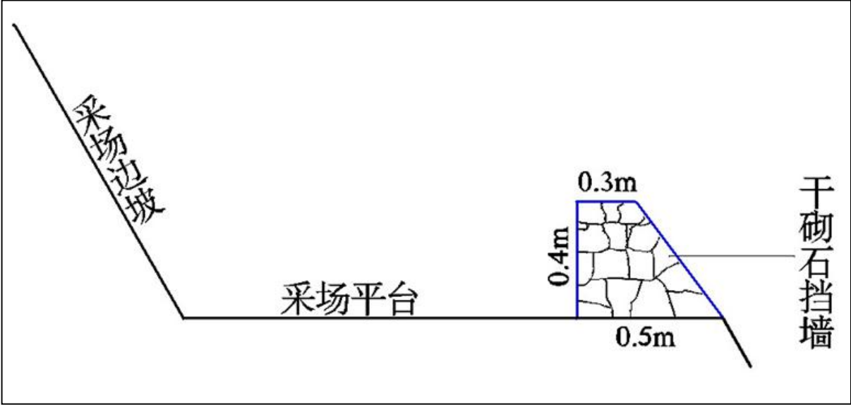
图 5-5 干砌石挡墙设计大样图
