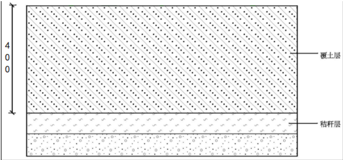
图 5-4 露天基底复垦设计图
