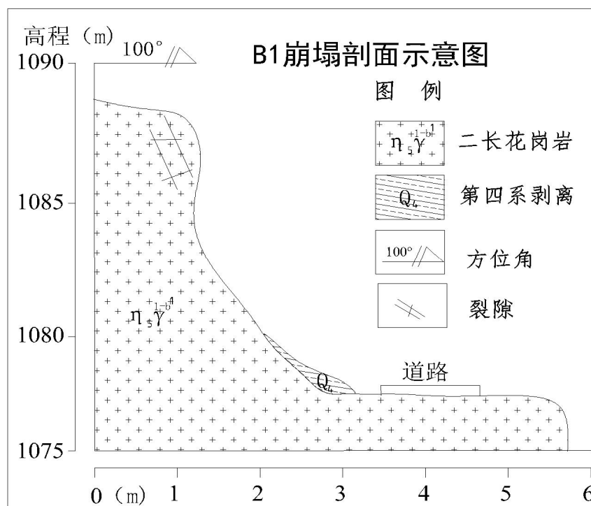
图 3-1 B1 崩塌剖面图
